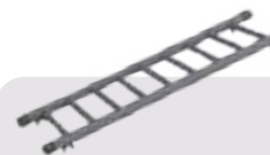
842533 長階梯 產品尺寸：1055 x 355 x 75h mm
